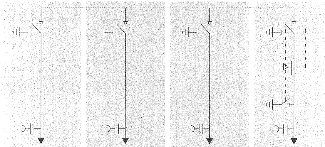
Фиг. 10 - Комплектна разпределителна уредба с SF 6 товари прекъсвачи – три кабелни присъединения и едно трансформаторно присъединение - КККТ
