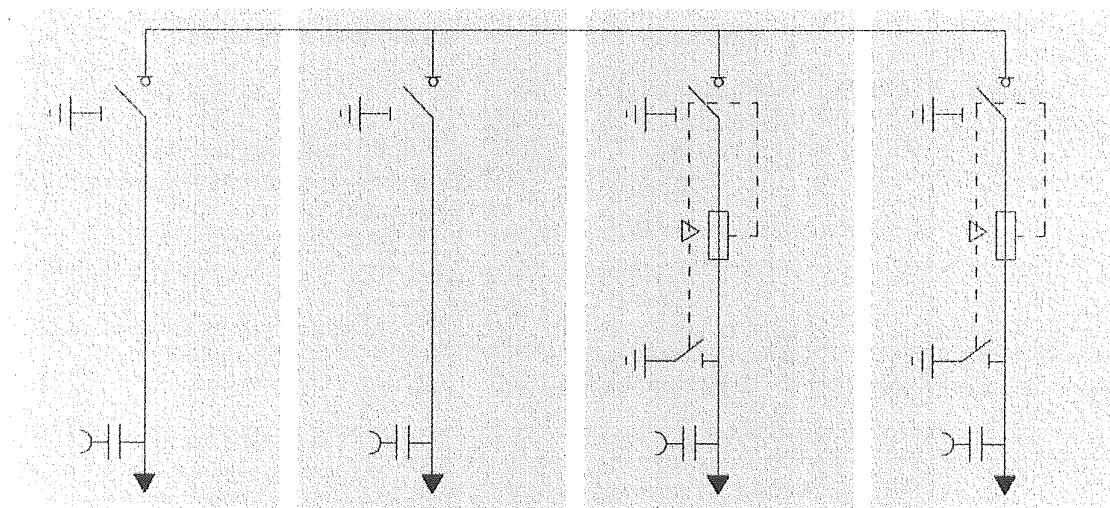
Фиг. 12 - Комплектна разпределителна уредба с SF 6 товари прекъсвачи – две кабелни присъединения и две трансформаторни присъединения – ККТТ
