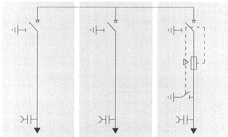
Фиг. 8 - Комплектна разпределителна уредба с SF 6 товари прекъсвачи – две кабелни присъединения и едно трансформаторно присъединение - ККТ
