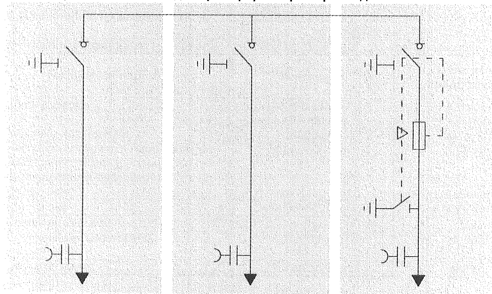
Фиг. 7 - Комплектна разпределителна уредба с SF 6 товари прекъсвачи – две кабелни присъединения и едно трансформаторно присъединение – KKT
